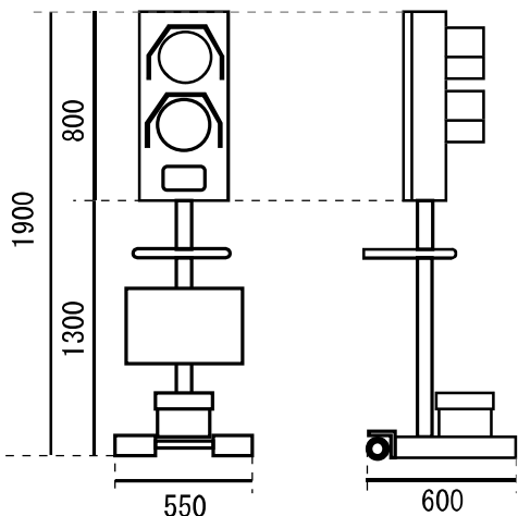
寸法図
